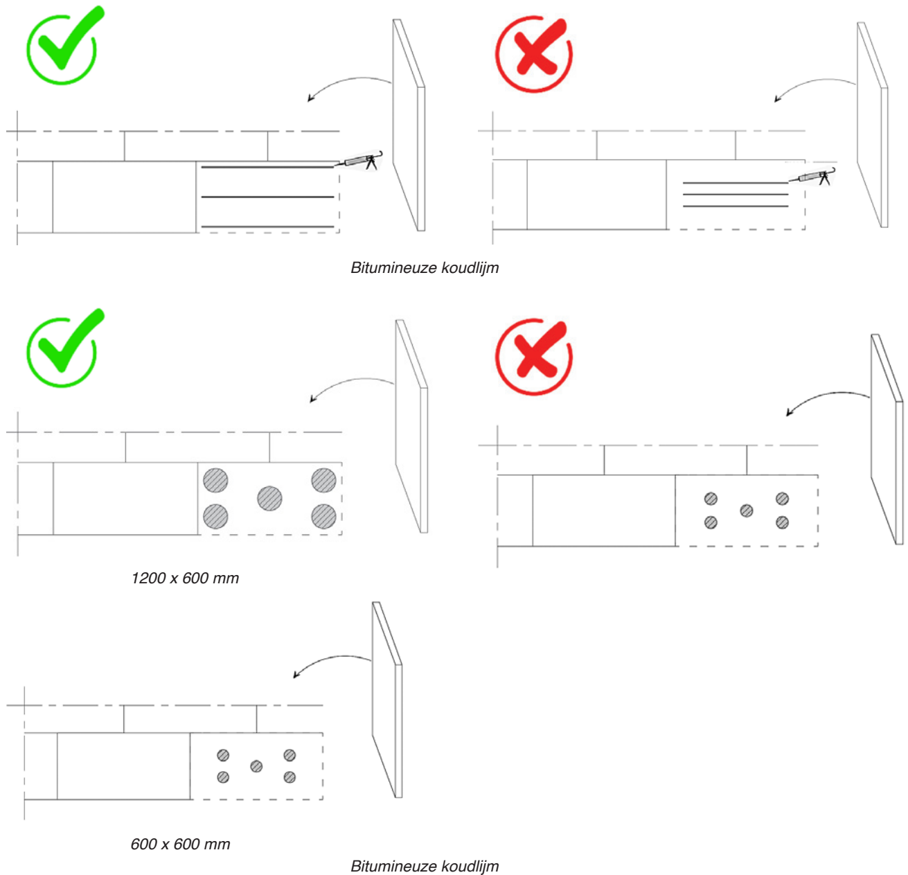
Figuur 7: Verkleefde opbouw - Lijmpatroon - bitumineuze koudlijm (principetekeningen 4 )
