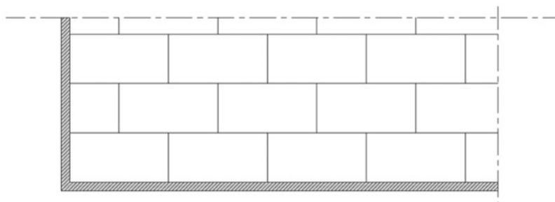
Figuur 4: Verspringend patroon binnen één enkele isolatielaag
