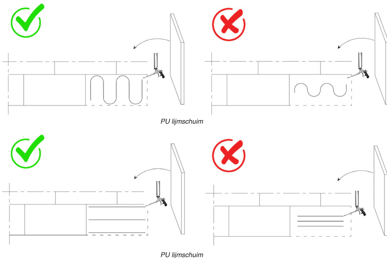
Figuur 6: Verkleefde opbouw - Lijmpatroon - PU-lijmschuim (principetekeningen 3 )
