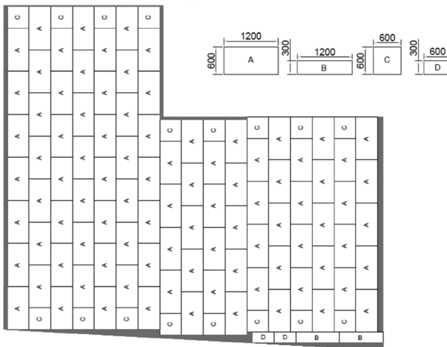
Figuur 2: voorbeeld van een legplan met aanduiding van de verschillende paneelformaten en de zones die dienen opgevuld te worden (grijs)
