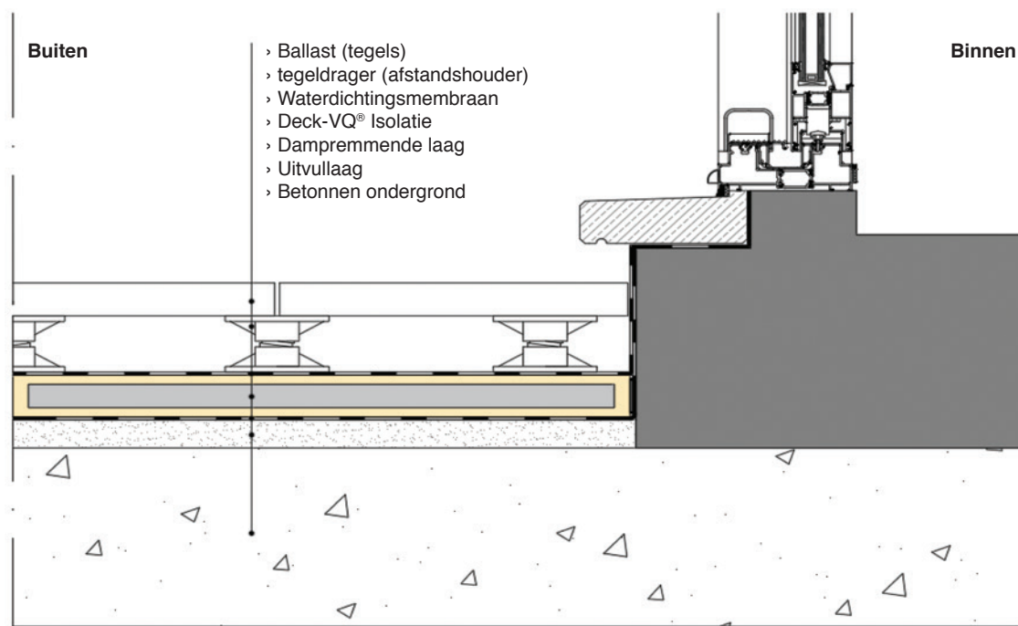
Figuur 9: Voorbeeld van een opbouw met ballast
