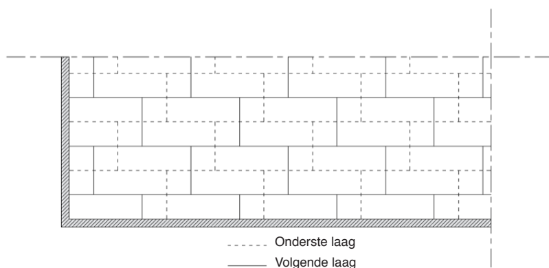
Figuur 5: Verspringend patroon in meerlaagse opbouwen
